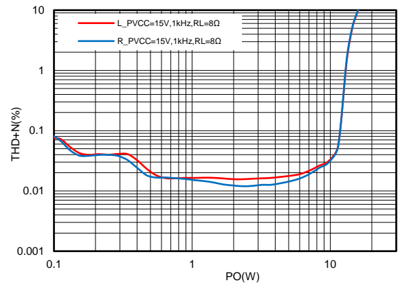
图19. 15V供电8Ω负载THD+N曲线BTL
