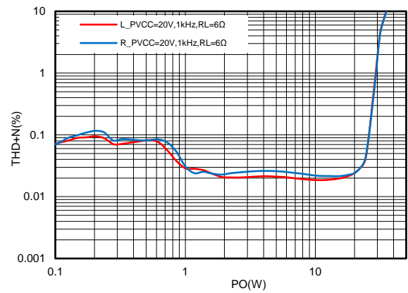
图17. 20V供电6Ω负载THD+N曲线BTL
