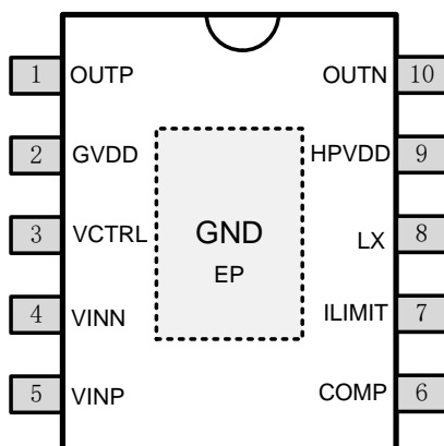
ESOP-10
