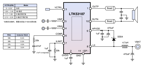
图1 LTK53107应用原理图
