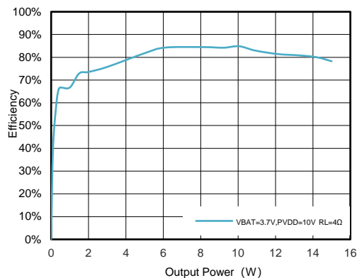
图10 Class D输出功率和效率
