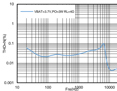
图8 3W功率下Class D频率和THD+N
