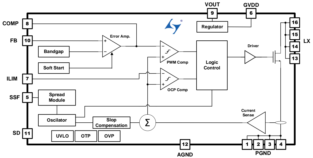
图3 LTK61103模块功能框图
