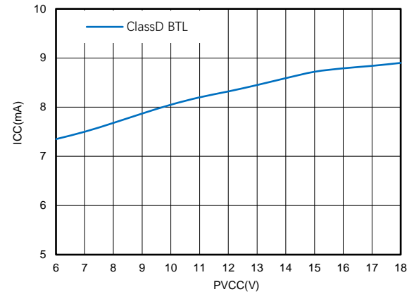
图23. 不同供电电压下的静态电流
